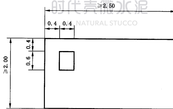
图 C.1 试验模型尺寸
