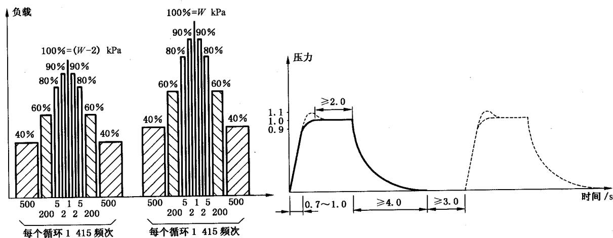
图 A.1 加压过程和压力脉冲示意图
