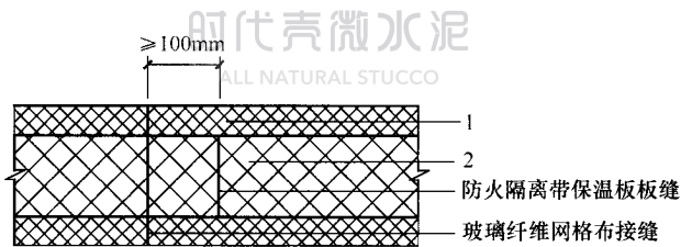
图 5.0.7-2 防火隔离带网格布水平方向对接
