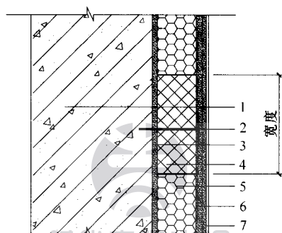
图 5.0.1 防火隔离带基本构造
