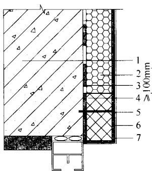
图 5.0.9 门窗洞口上部 防火隔离带做法（一）
