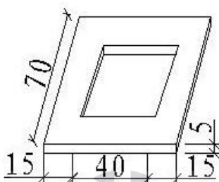
图1 橡胶或硅酮密封材料制成的成型模框
