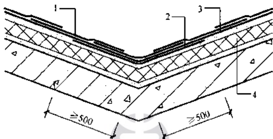
图 4.11.13 沥青瓦屋面天沟
