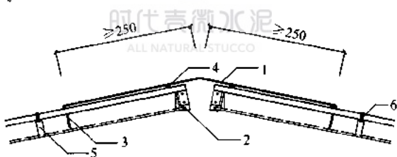
图 4.11.28 金属板材屋面屋脊
