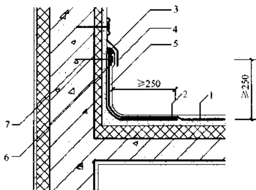
图 4.11.14-2 高女儿墙
