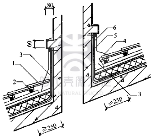
图 4.11.20 烧结瓦、混凝土瓦屋面烟囱
