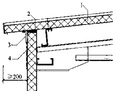
图 4.11.10 金属板屋面檐口
