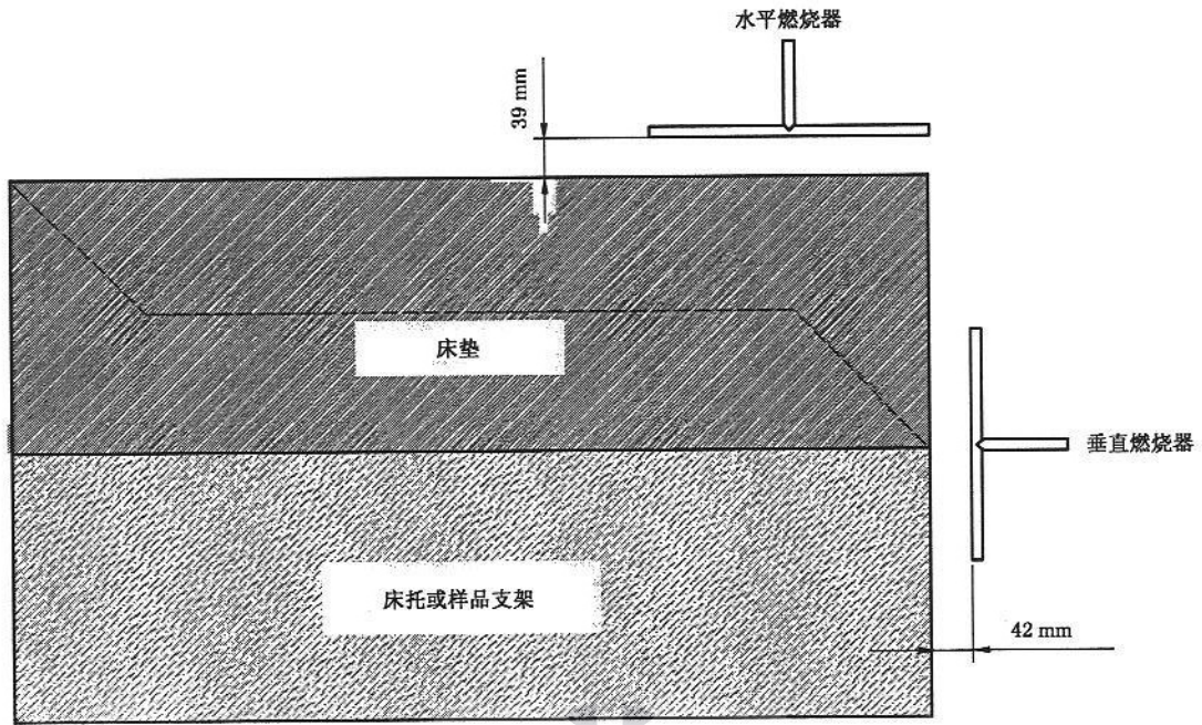
a) 侧视图
